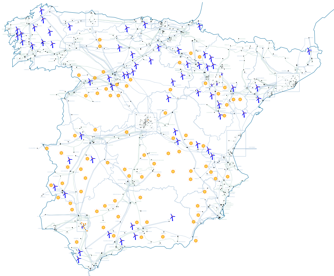
Figura 5. Ubicación de nueva generación renovable en el escenario de estudio. Sistema peninsular
